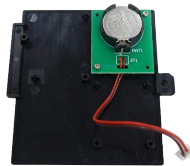
RTC module
